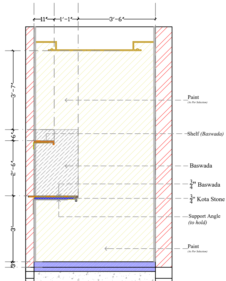
ELEVATION B
