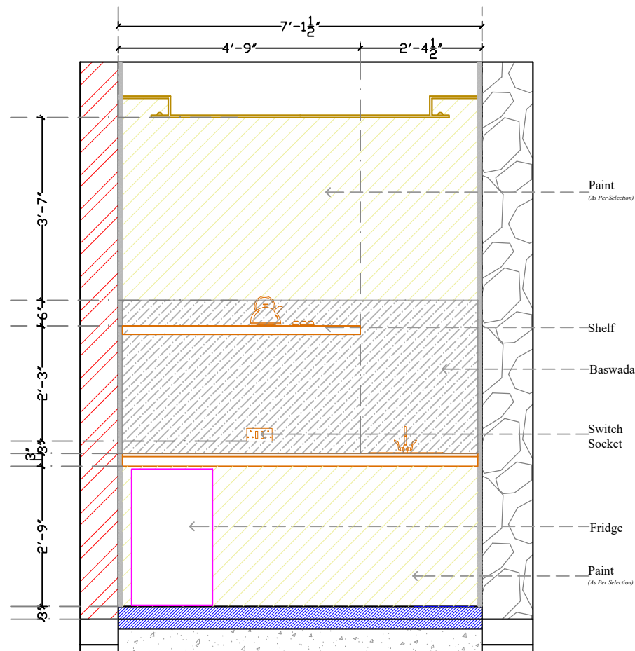
ELEVATION A
