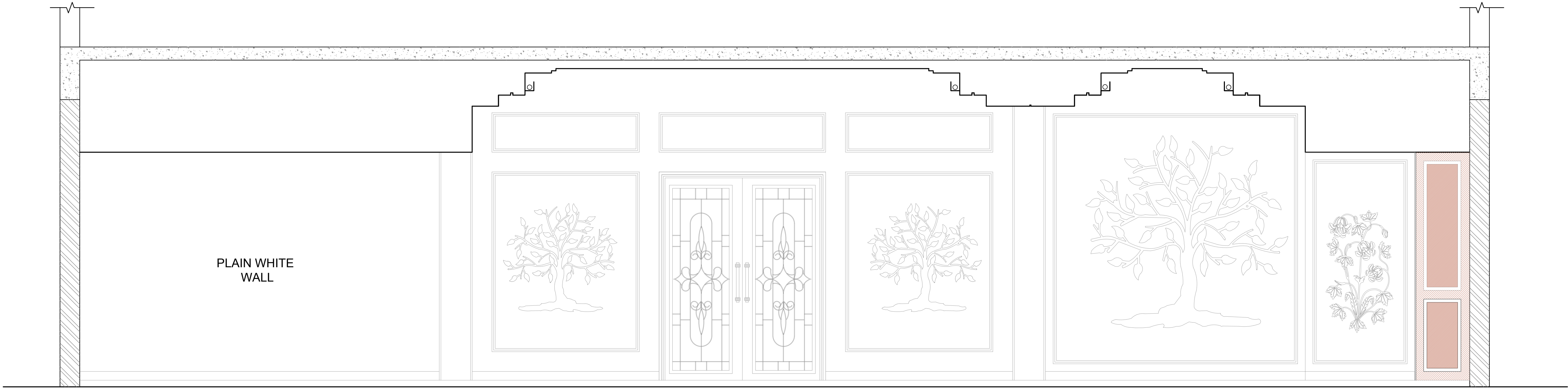
ELEVATION A
