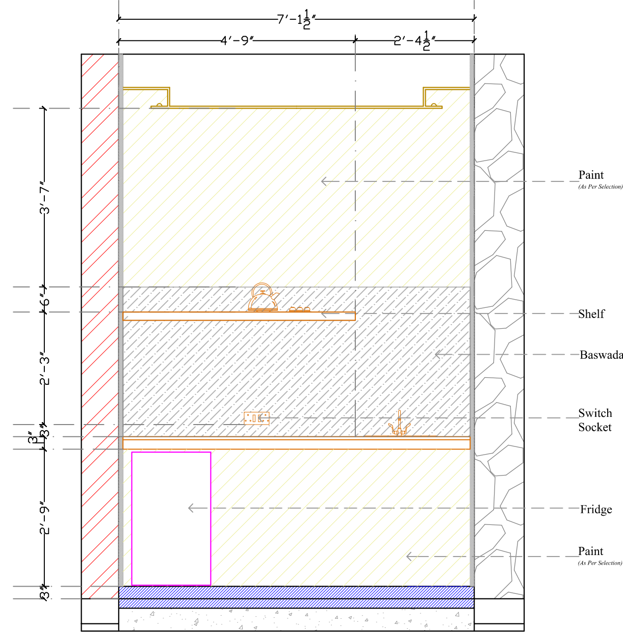
ELEVATION A
