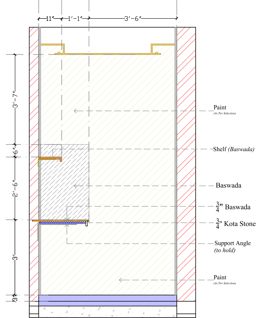
ELEVATION B
