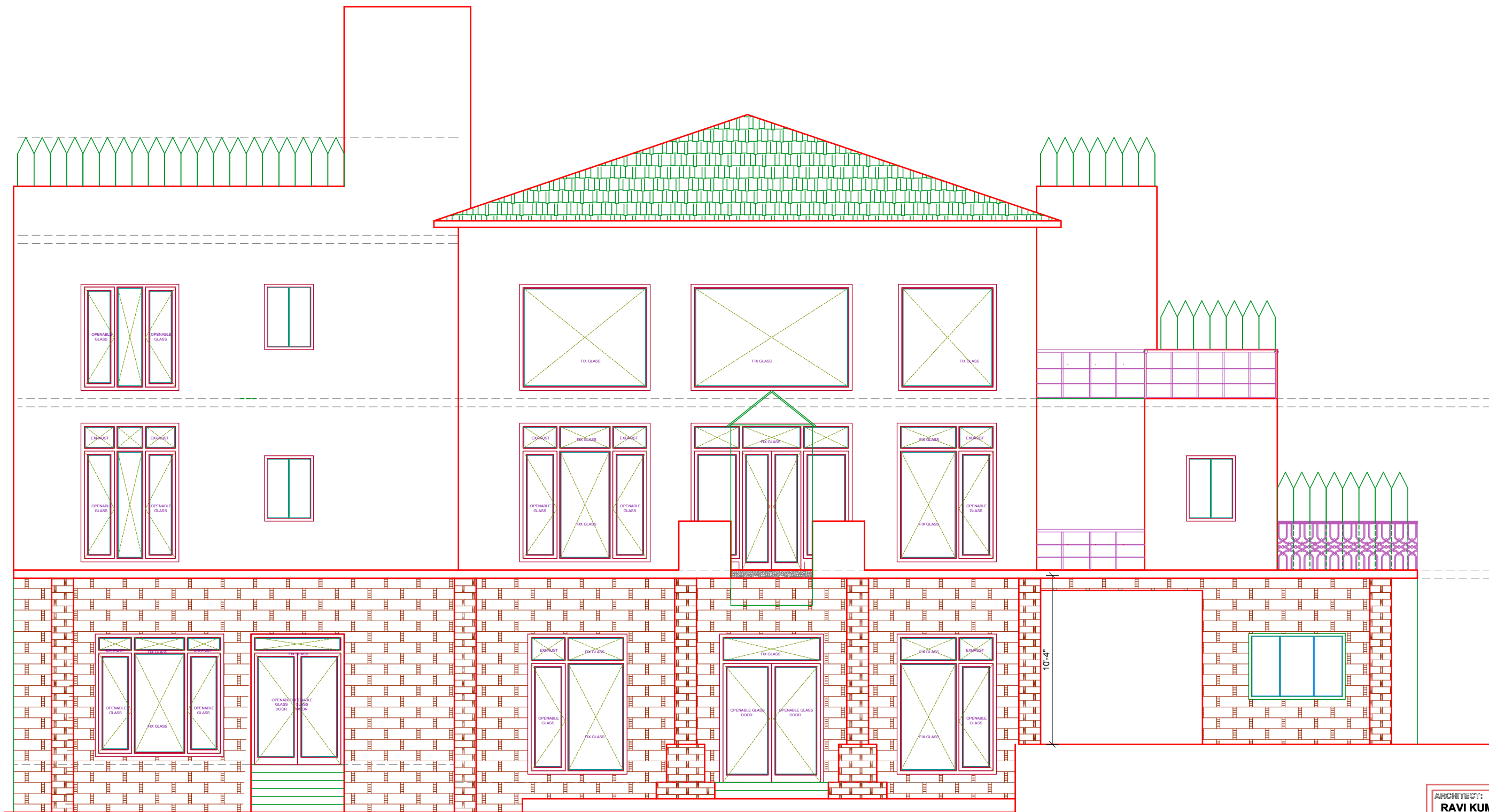
ELEVATION
