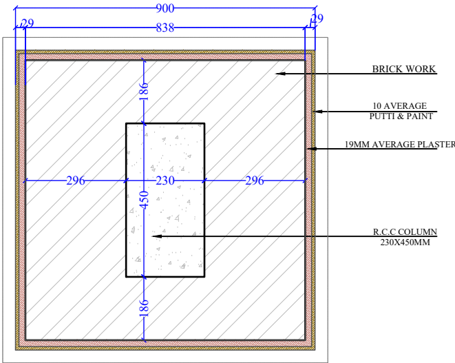
SECTION A4
