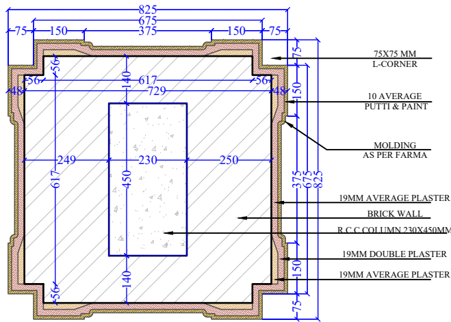
SECTION A3
