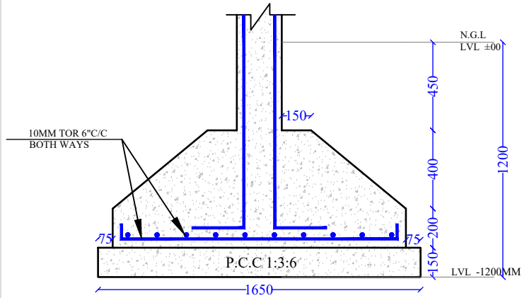
SECTION 1-1 (F1)
