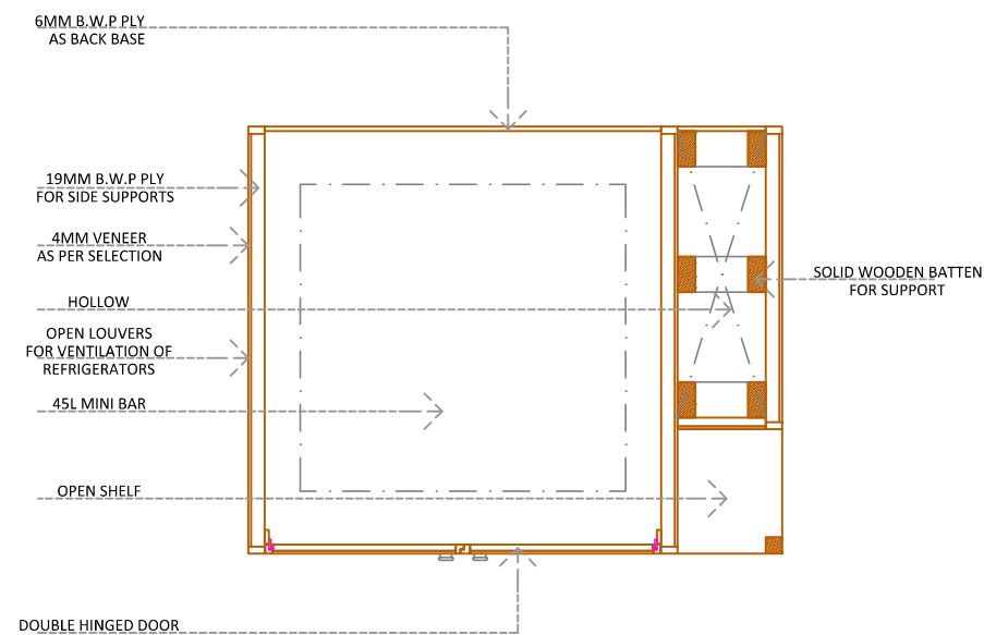
PLAN: MINI BAR
