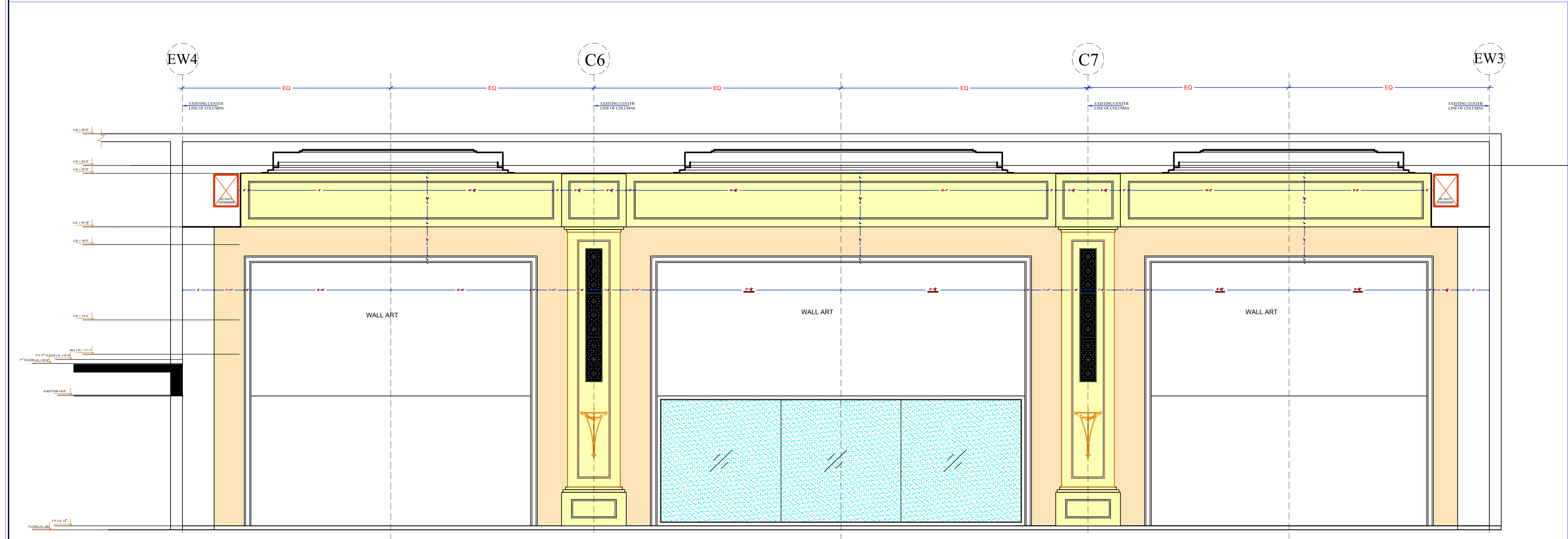
ELEVATION B
