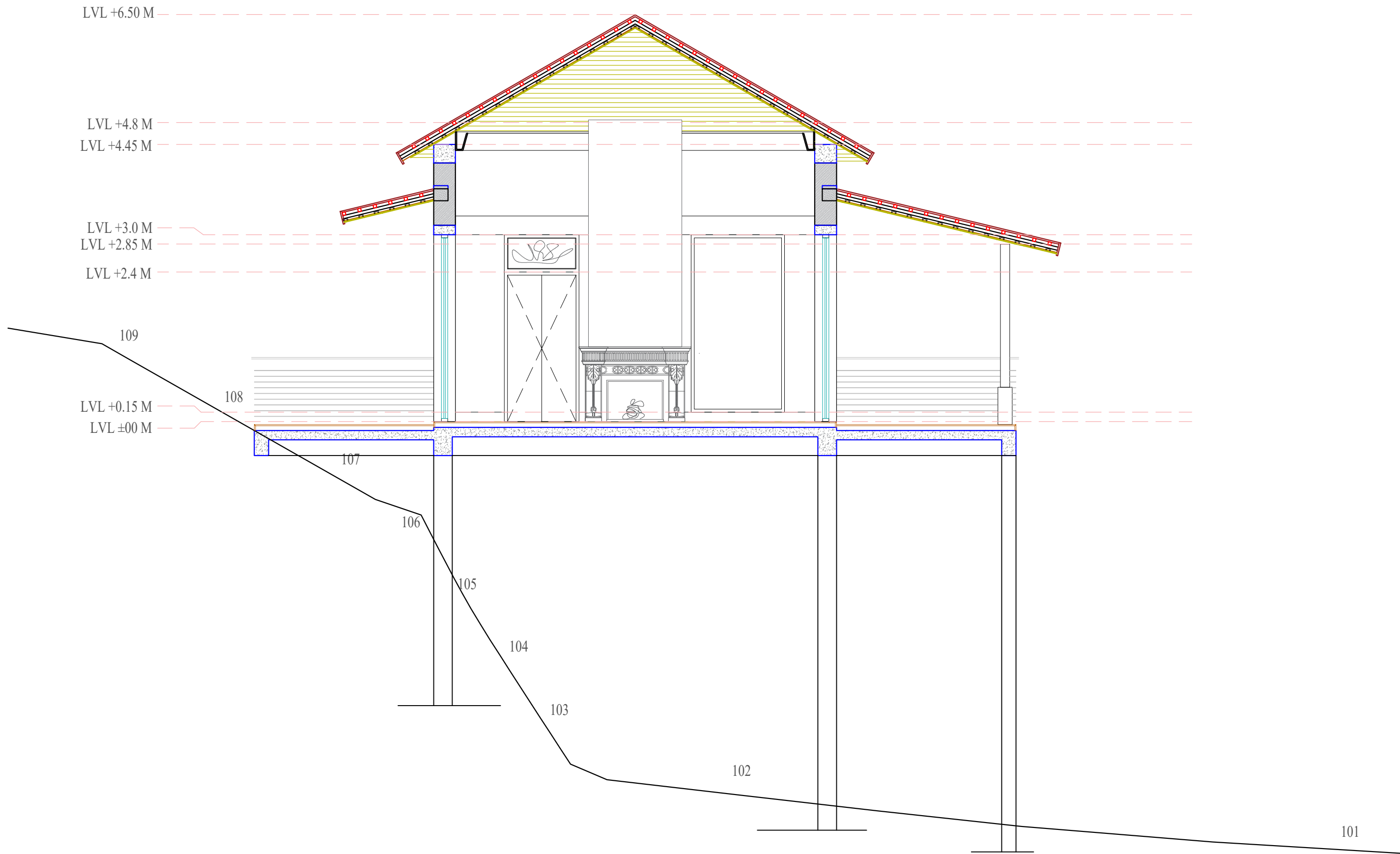
Section EE(bedroom)
