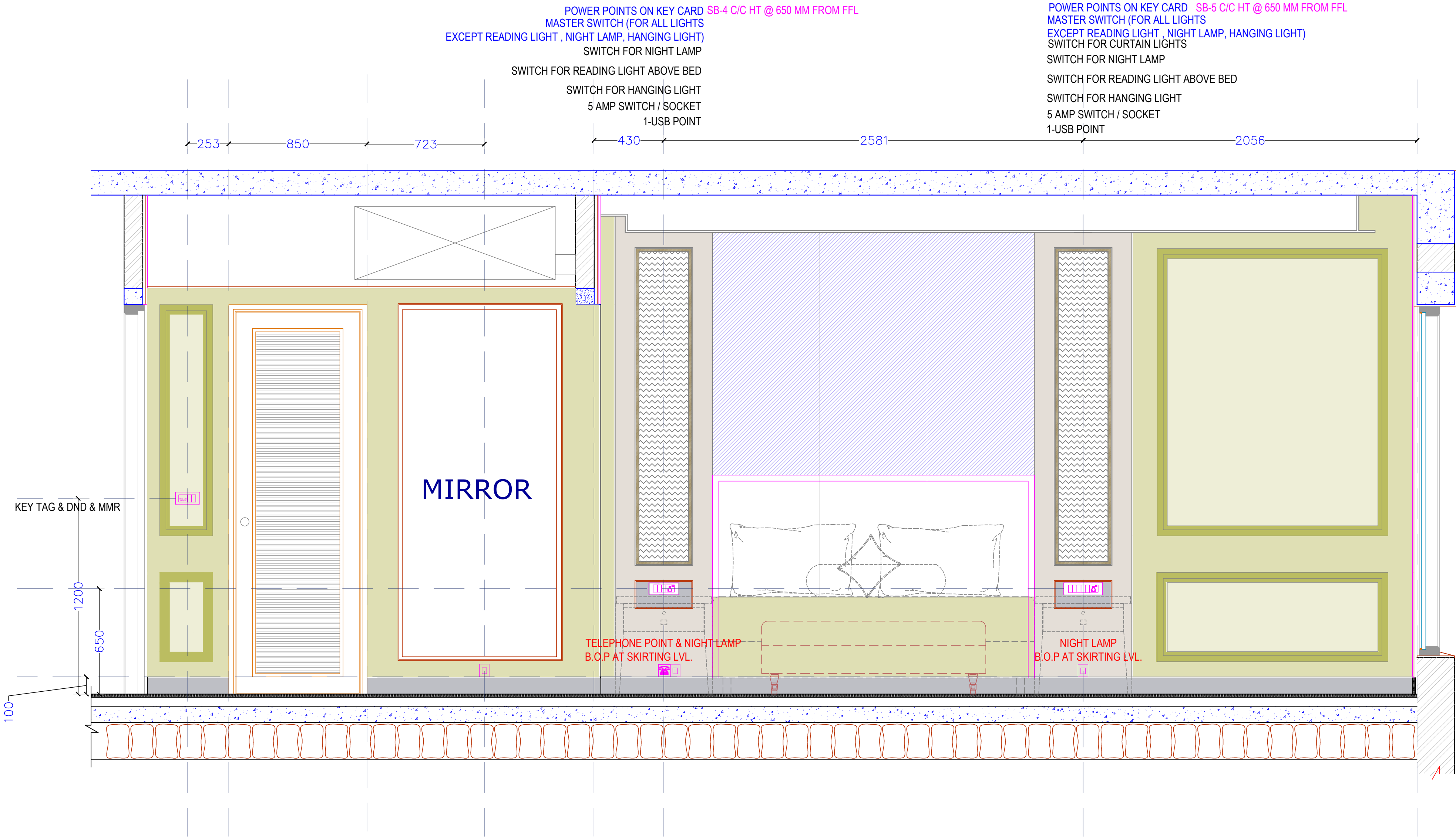
ELEVATION A
