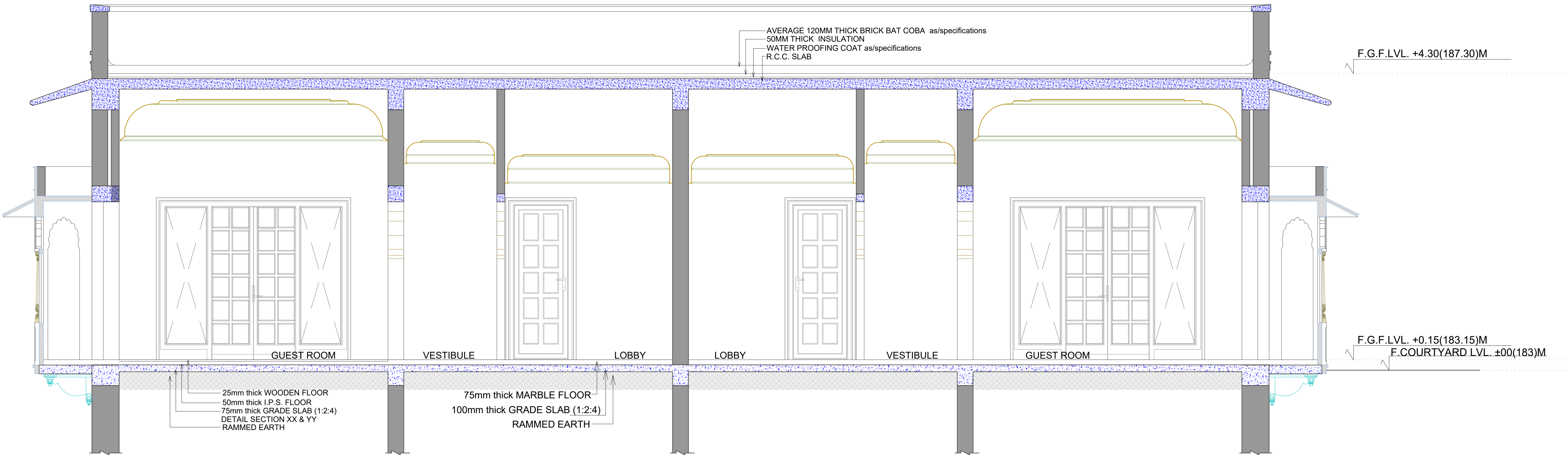
SECTION A-A
