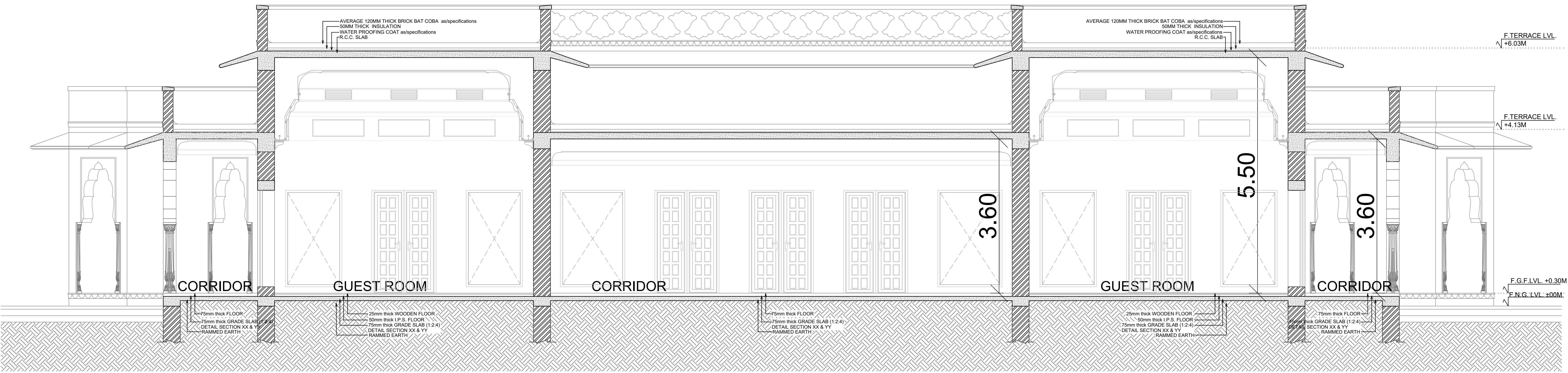
SECTION A-A
